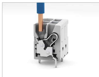
単線またはフェルール圧着線は差し込みだけのプッシュ・イン結線
