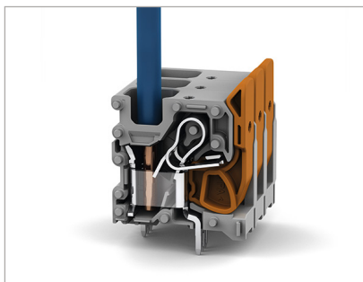
単線またはフェルール圧着線は差し込むだけのプッシュ・イン結線
