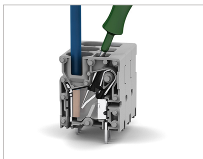
より線はドライバ操作で簡単結線
