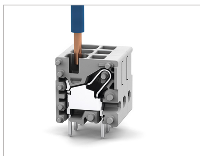
単線またはフェール圧着線は差し込むだけのプッシュ・イン結線
