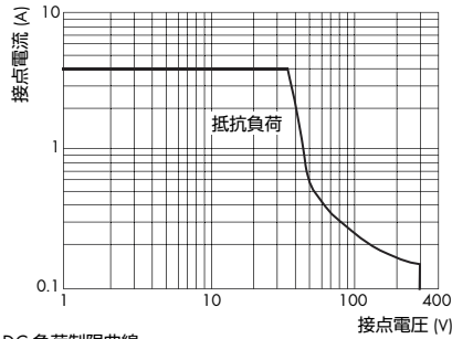
DC 負荷制限線
