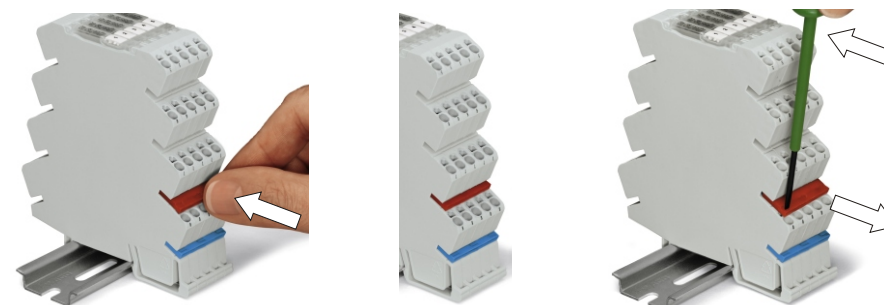
完全に固定するまで差込型ジャンパを押し込む
