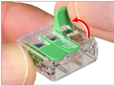
①レバーを押し上げます。
