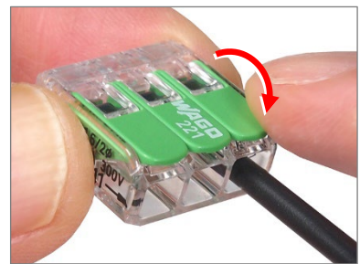
③レバーを押し下げれば、結線の完了です。
