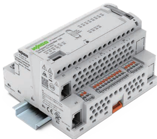
電源電圧 (フィールド) デジタル入力 (PNP) RTD 入力 アナログ入力 microSD カードスロット USB-C フィールドバス接続 2 x RJ-45 電源電圧 (フィールド) 電源電圧 (システム) アナログ出力 デジタル出力 (PNP)
